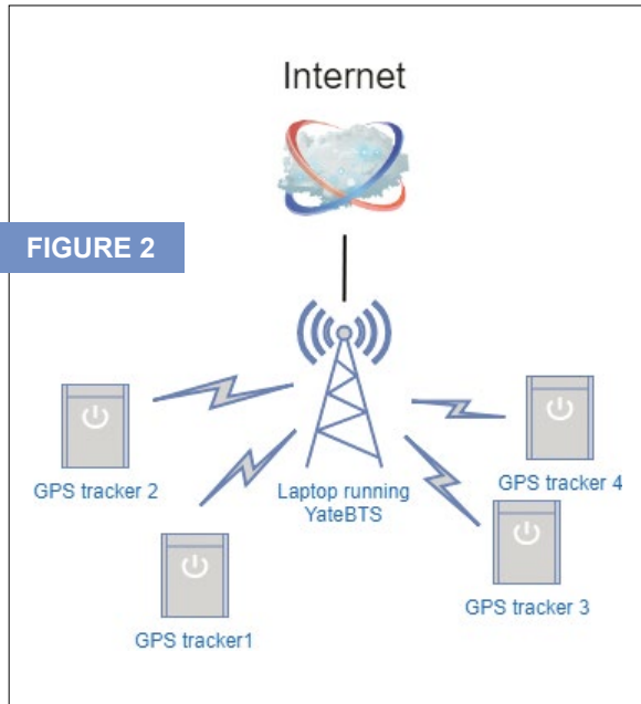
Mise en place d'un BTS permettant l'interception des flux réseaux en 2/2.5G.
