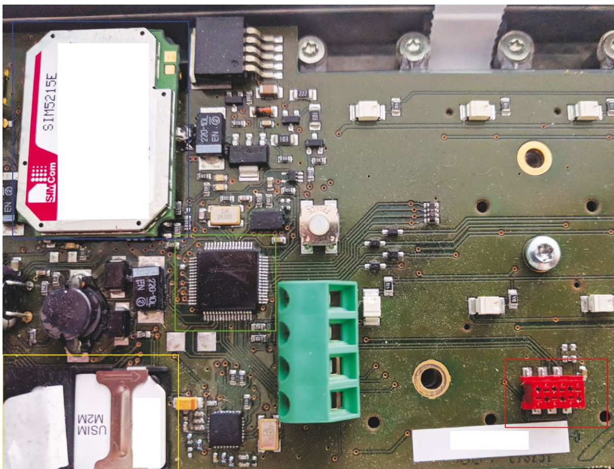
FIGURE 7 Composants d'un interphone connecté.
