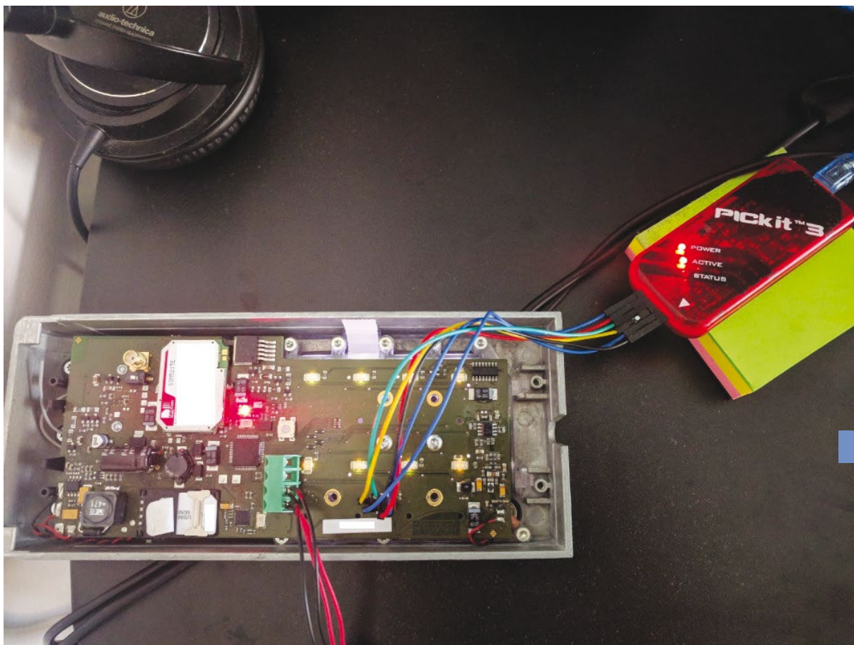
Utilisation du Pickit3 pour les microcontrôleurs PIC.
