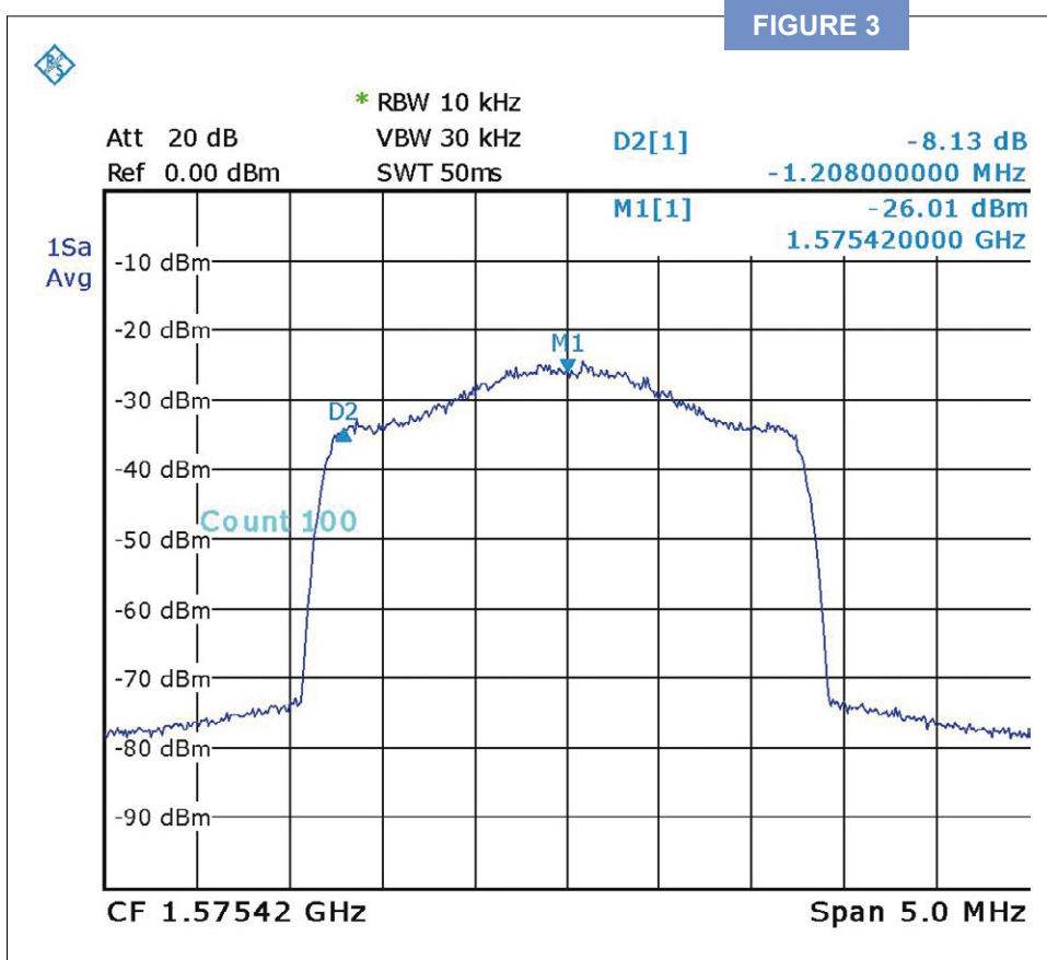
Spectre du signal émis par la PlutoSDR réglée sur un gain de 0 dB : la porteuse à 1575,42 MHz est étalée spectralement sur \pm 1 \text{ MHz} par modulation en phase selon la séquence pseudo-aléatoire caractéristique de chaque satellite, induisant un niveau de -30 dBm environ dans la bande.
