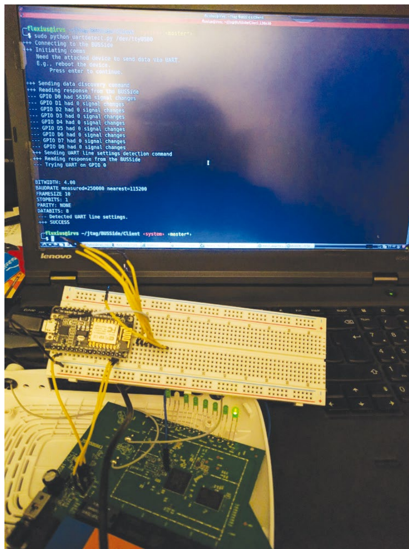
FIGURE 12 Utilisation du BUSSide avec un ESP8266 pour bruteforcer les pins JTAG et UART.
