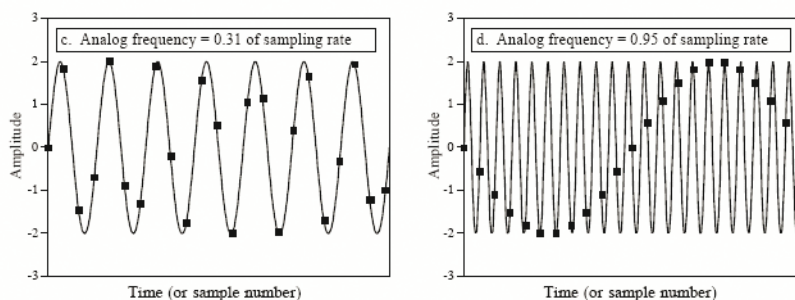
Fig. 5 : Résultat d'un « aliasing » lorsque la fréquence d'échantillonnage est trop faible (source : DSPGUIDE [49]).
