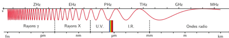
Fig. 2 : Domaine de spectre des ondes électromagnétiques (source : Wikipédia).
