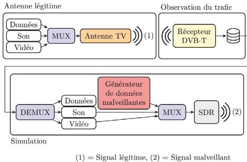
Fig. 2 : La plateforme d'émission DVB-T.
