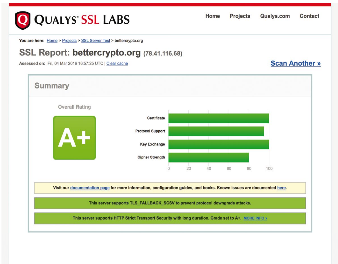
Fig. 3 : SSL Labs sur BetterCrypto.org.
