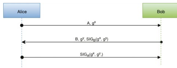
Fig. 3 : Diffie-Hellman authentifié.
