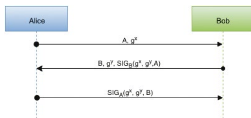
Fig. 5 : Échange de clefs de type ISO-9796.
