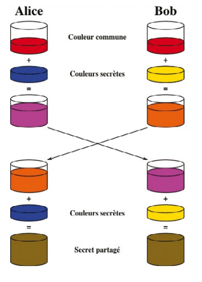
Fig. 2 : Échange Diffie-Hellman avec de la peinture.
