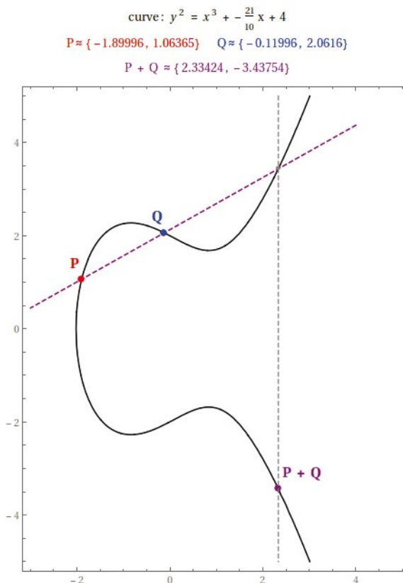
Fig. 1 : Représentation d'une courbe elliptique et addition géométrique de 2 points.
