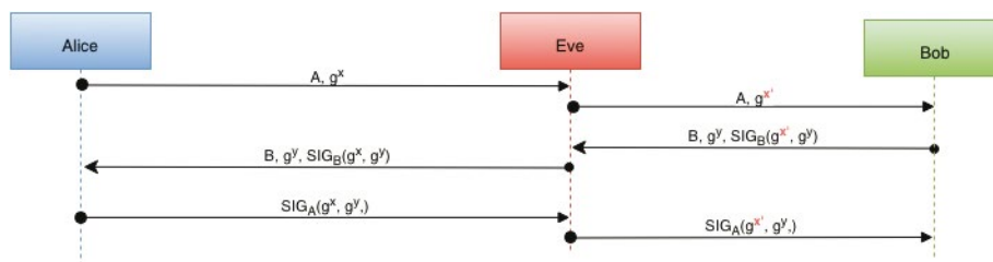
Fig. 6 : Attaque de type replay avec un x fixé.
