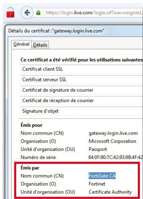
Fig. 10 : Client intercepté par Fortigate240D.
