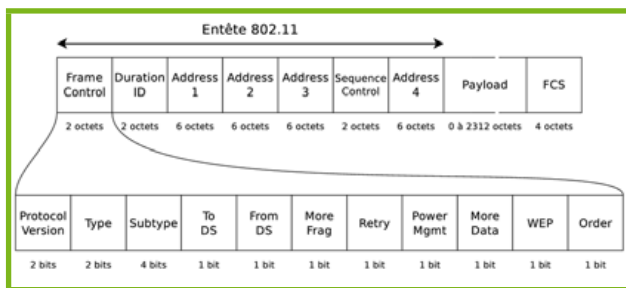
Fig. 2 : Décomposition d'une trame 802.11 et du champ Frame Control
