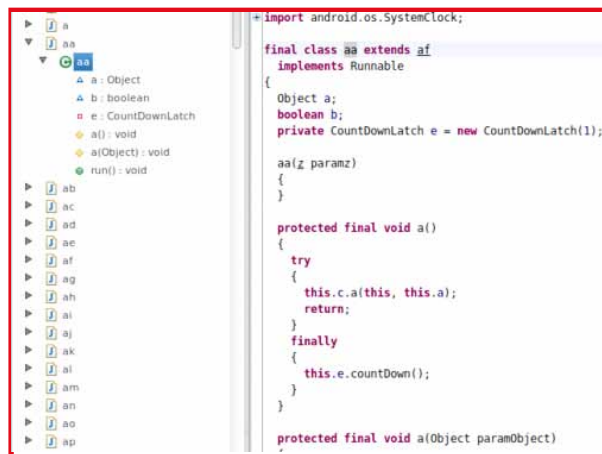
Fig. 1 : Exemple d'application obfusquée par Proguard
