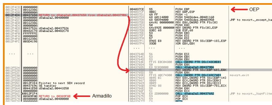
Fig. 3 : Entry point d'un malware compilé avec VisualStudio et lié dynamiquement, reconnaissable grâce à la signature 558BEC6AFF68????68????64A1000000050648925000000083EC685356578965E833DB895DFC6A02FF15
