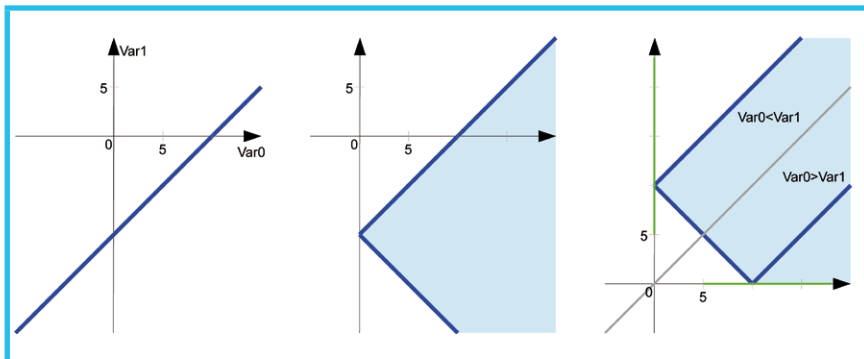
Fig.2 : Ensemble des couples (Var0,Var1) possibles aux lignes 3, 5, et 7. Les lignes bleues représentent l'ensemble exact, la zone bleue claire représente une approximation par un polyèdre convexe.
