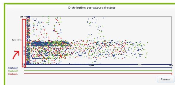
Fig. 2 : Affichage dans l'interface graphique de Netzob de la distribution des valeurs pour chaque octet sur les 3 sessions. La flèche rouge désigne une zone de données à faible entropie.
