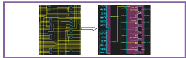
Fig. 5 : Abstraction fonctionnelle
