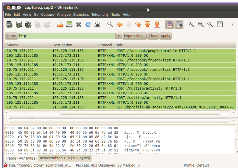
Fig. 1 : Extrait de la capture réalisée sous Wireshark
