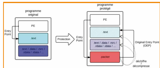
Fig. 1 : Schéma simplifié du fonctionnement général d'un packer et illustrant les deux étapes de la protection.
