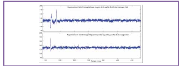
Fig. 7 : Rayonnement électromagnétique moyen de la manipulation de la partie droite et de la partie gauche du message clair par un crypto-système
