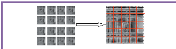
Fig. 3 : Recalage pyramidal
