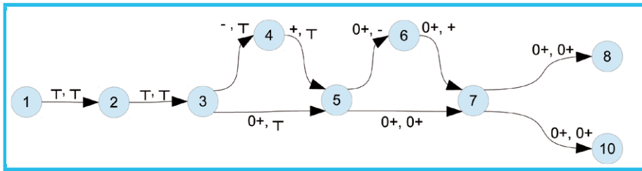
Fig.1 : Valeur abstraite de (Var0,Var1) sur le programme \max(|Arg|, |Arg-10|)
