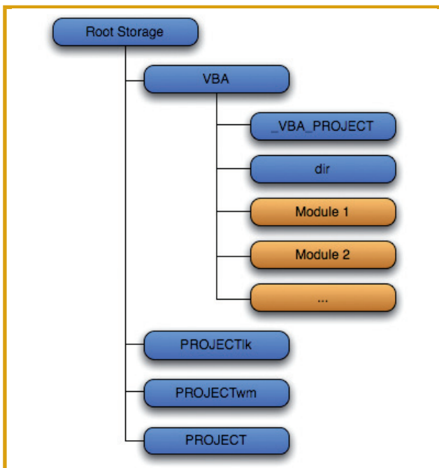
Figure 5 - Structure d'un storage VBA
