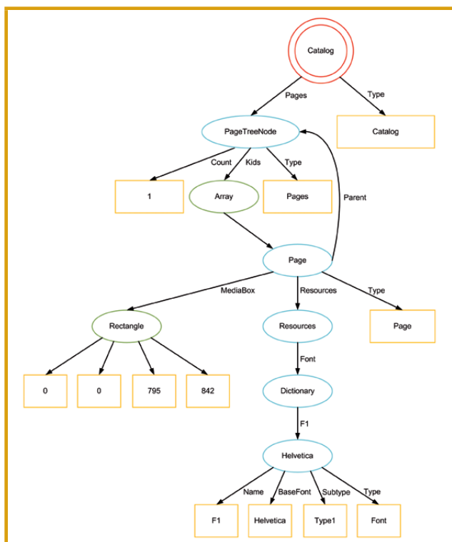
Figure 3 - Graphe du PDF 'blanc' généré par défaut par Origami
