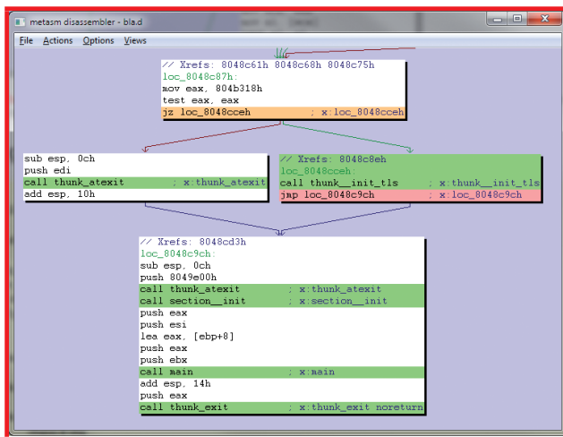
Coloration syntaxique
