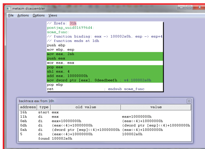
Backtracking illustré
