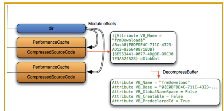
Figure 6 - Lecture d'une macro VBA
