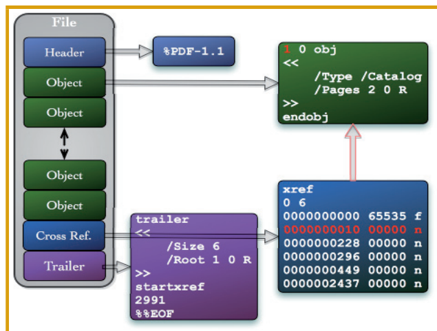
Figure 1 - Structure physique d'un fichier PDF
