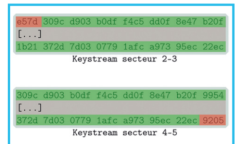
Fig. 3 : Décalage du keystream.
