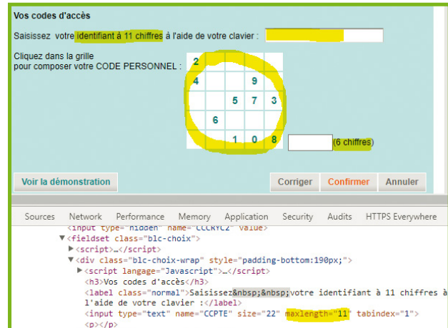
Fig. 2 : Pavé numérique aléatoire avec détails de la password policy.
