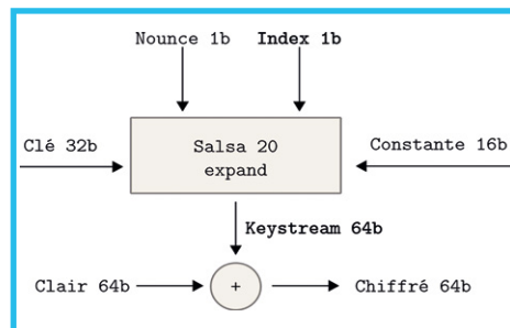
Fig. 2 : Chiffrement des données avec Salsa20.
