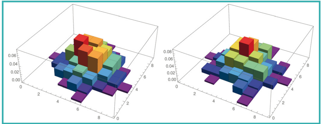
Fig. 3 : Distributions jointes de HW(X) et HW(Z) pour k_i = 39 (à gauche) et k_i = 167 (à droite).
