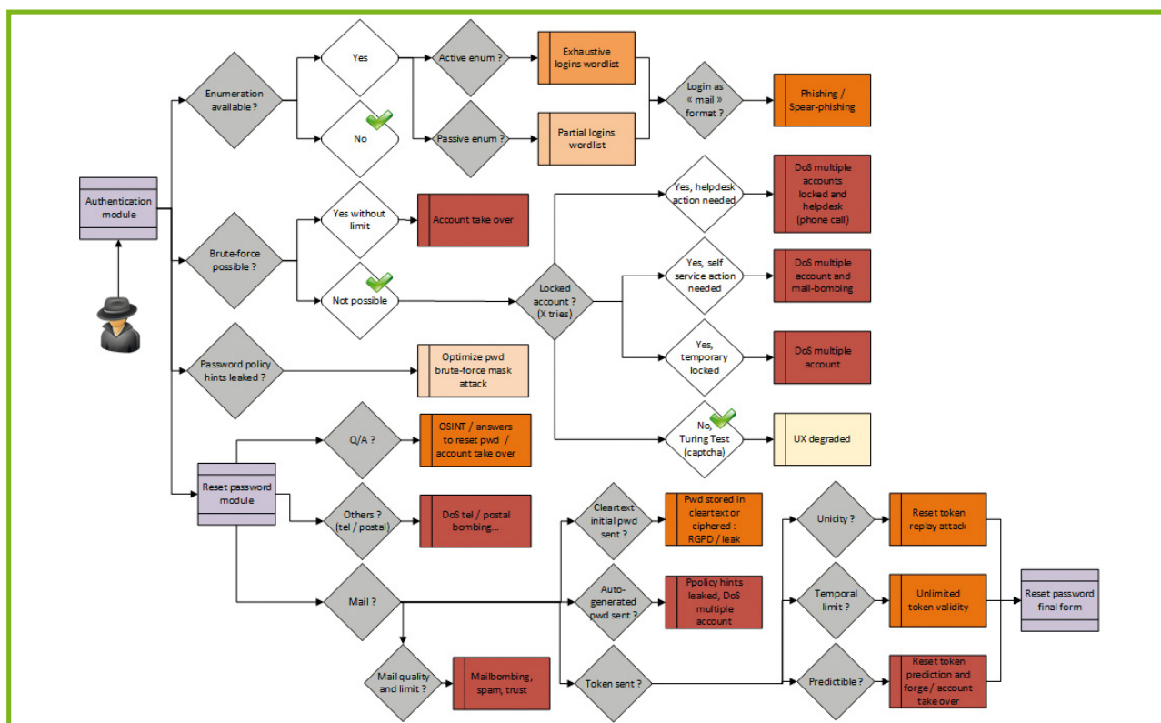
Fig. 3 : Arbre des faiblesses en fonction des approches fonctionnelles.
