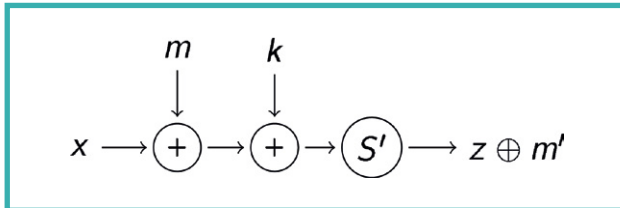
Fig. 1 : Addition de la clef et S-box masquées dans la première ronde de l'AES.
