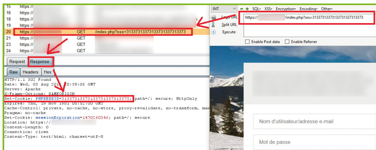
Fig. 1 : Illustration d'une session fixation attack rencontrée sur un bug bounty.
