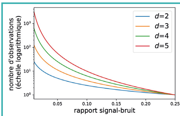
Fig. 2 : Évolution du nombre d'observations nécessaires pour attaquer une valeur masquée en fonction du rapport signal-bruit et de l'ordre de masquage.
