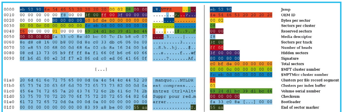
Figure 3 : Secteur de démarrage d'une partition NTFS.
