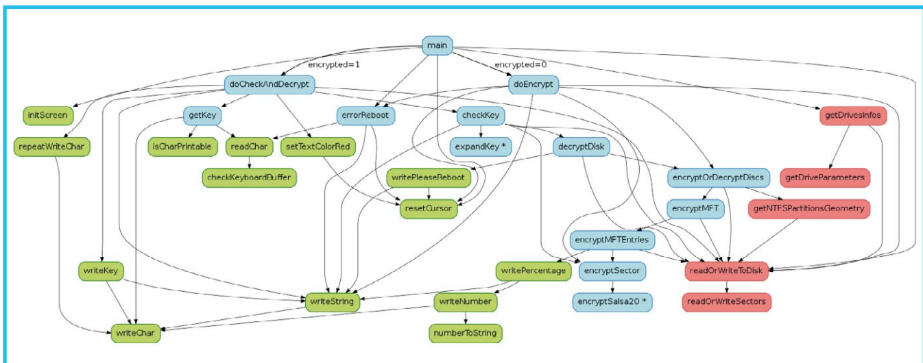
Figure 6 : Fonctionnement simplifié du code de démarrage de NotPetya.
