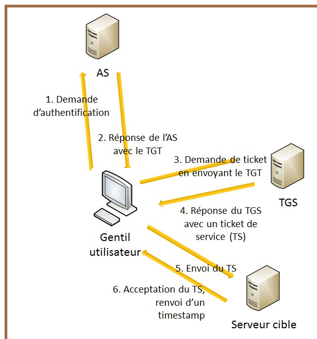
Figure 4 : Phase d'authentification Kerberos.
