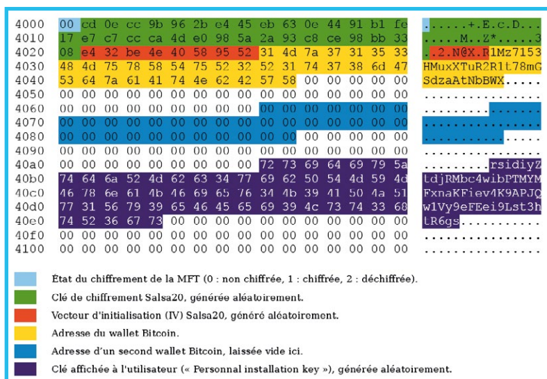
Figure 1 : Fichier de configuration de NotPetya.
