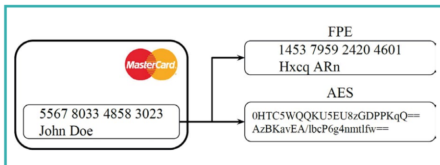
Figure 1 : Exemple de chiffrement d'une carte de crédit.
