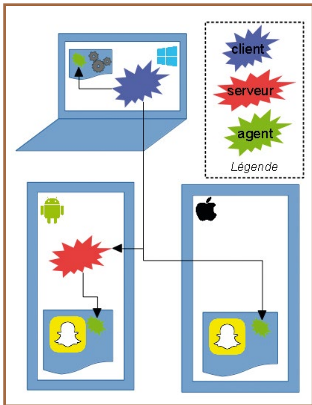
Fig. 1 : Schéma résumant les interactions entre les différentes briques de Frida.
