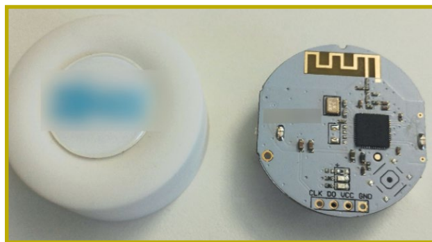
Fig. 4 : Accès hardware à une balise.
