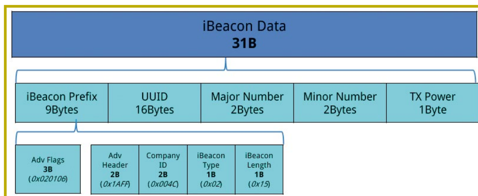
Fig. 1 : Format des paquets iBeacon.
