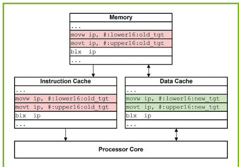
Fig. 1 : Caches de données et d'instructions des processeurs MIPS.
