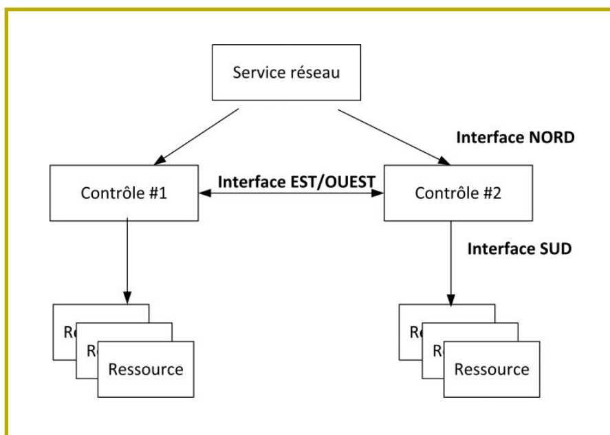
Figure 2 : Interfaces SDN pour le plan de contrôle.
