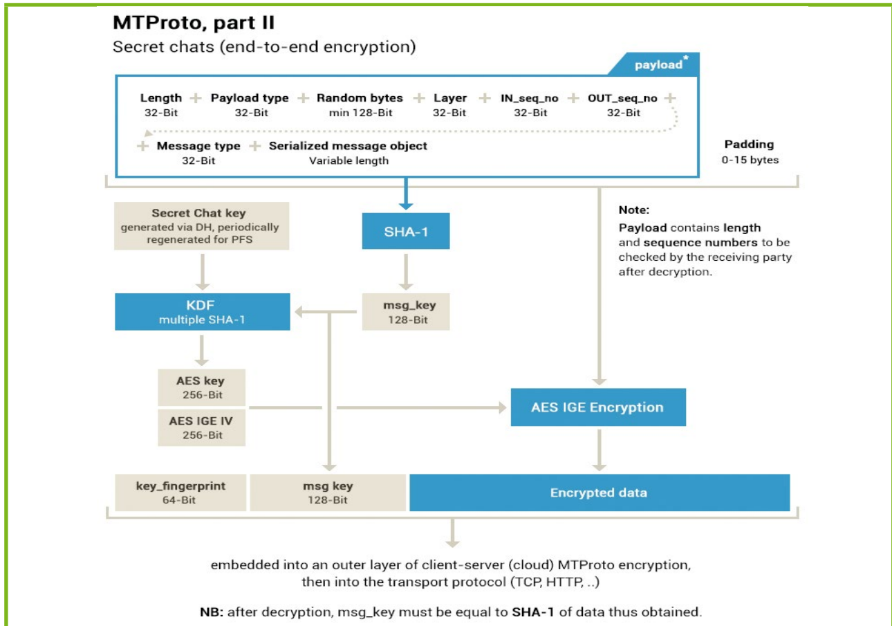
Figure 4 : Chiffrement des secret chats – documentation Telegram.
