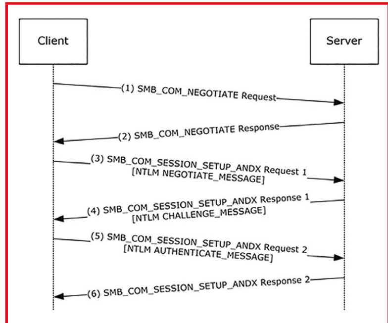
Figure 1 : Inclusion de l'authentification NTLM dans une session SMB.
