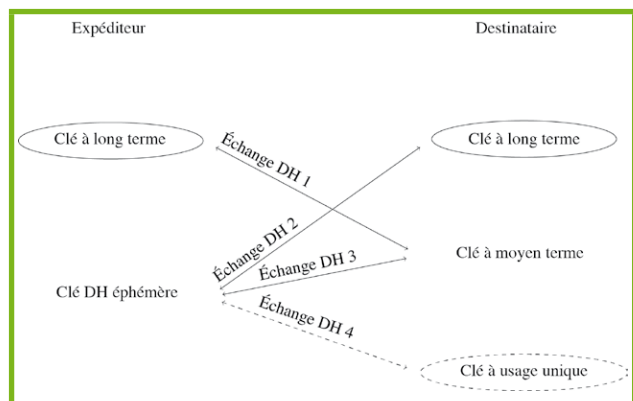
Figure 1 : Illustration des échanges de clés DH effectués dans le cadre de X3DH. Le trait en pointillés représente un échange optionnel, qui n'a lieu que si une clé à usage unique est disponible pour l'équipement destinataire.
