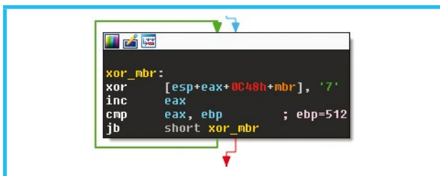
Figure 1 : XOR '7' appliqué au MBR.
