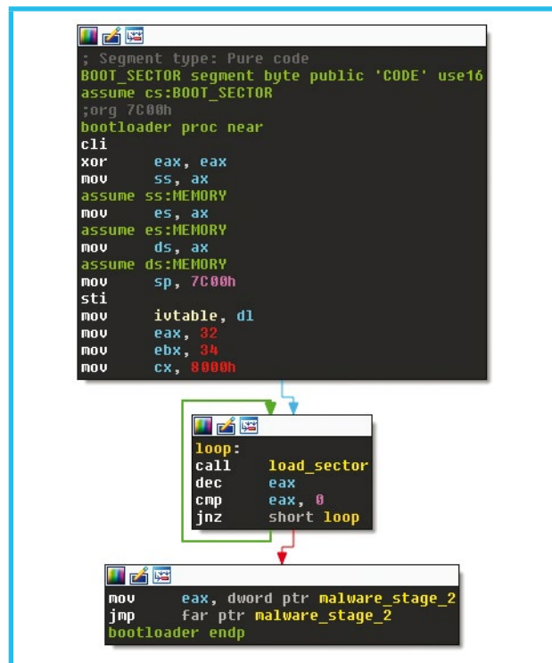
Figure 3 : Charge les secteurs en mémoire depuis le disque.
