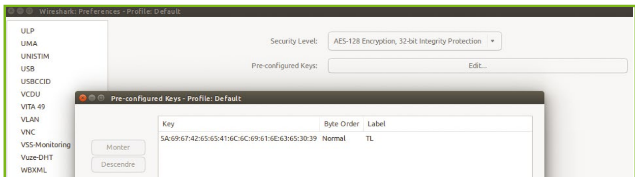
Figure 7 : Ajout de la Link Key du Trust Center dans Wireshark.
