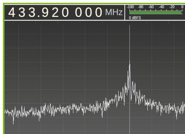
Figure 1 : Pic de fréquence à 433,92 Mhz.
