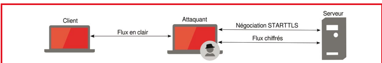
Figure 5 : Schéma d'une attaque classique de Downgrade STARTTLS.
