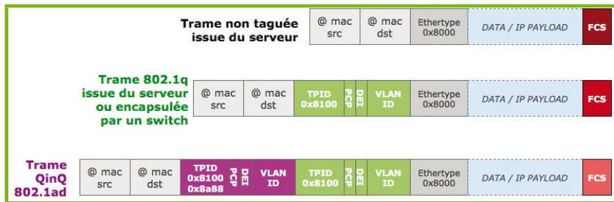
Figure 1 : Ajout des tags 802.1q et 802.1ad à une trame Ethernet.
