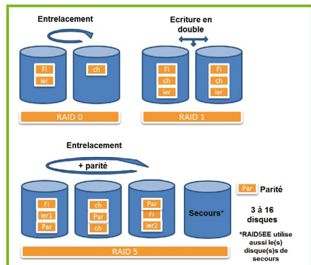
Figure 1 : Modes RAID les plus courants.
