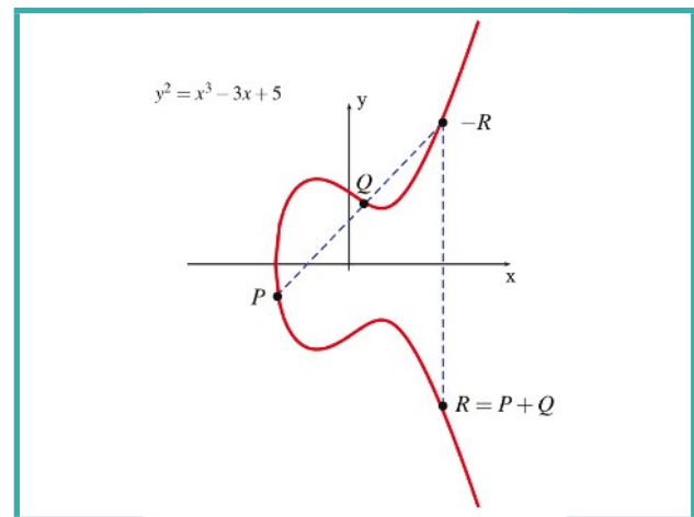
Figure 4 : Addition dans le corps associé sur une courbe elliptique.
