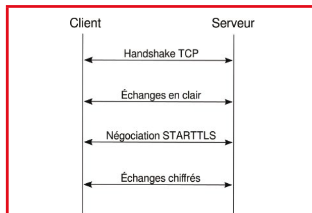
Figure 3 : Négociation STARTTLS au cours d'une communication.
