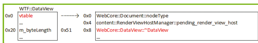
Fig. 7 : WTF::DataView.
