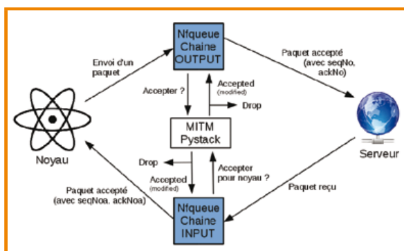
Fig.4 : Schéma global du fonctionnement de l'attaque de MITM.
