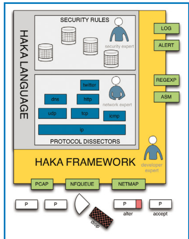
Fig. 1 : Architecture de Haka.
