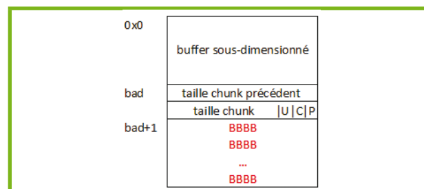
Fig. 1 : ArrayBuffer alloué à la suite du buffer sous-dimensionné.
