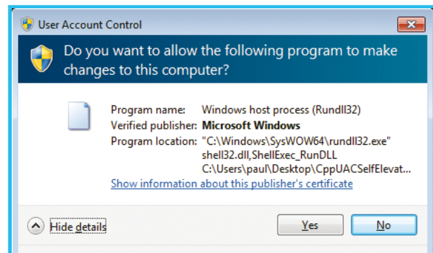
Fig. 7 : Détail de la fenêtre UAC lors de l'exécution d'une commande via rundll32.exe.
