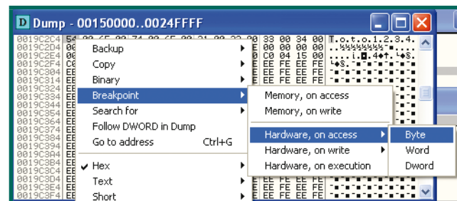
Fig. 3 : Ajout du HBP en accès sur le mot de passe.
