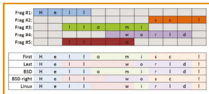
Fig.2 : Exemple du résultat du réassemblage d'une chaîne de caractères en fonction de la stratégie employée.
