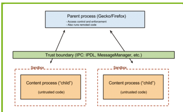
Fig. 1 : Modèle multiprocessus de Firefox OS.
