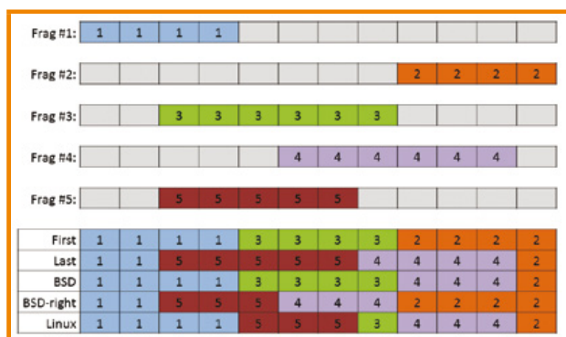
Fig. 1 : Réassemblage de 5 fragments IP en fonction de la stratégie de réassemblage. Les numéros indiquent l'origine de la donnée en considérant que les fragments sont envoyés dans l'ordre Frag #1, #2...
