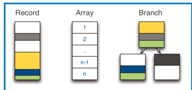
Fig. 2 : Grammaire Haka – Éléments composés.
