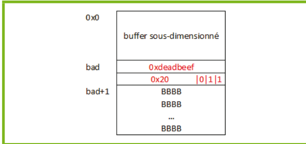
Fig. 2 : Modification des métadonnées du tas.
