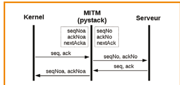
Fig. 3 : Schéma simple de la gestion des numéros de séquence, acquittement et prochain numéro de séquence tels qu'utilisés pour l'attaque de MITM.
