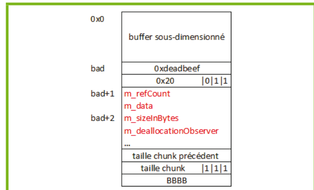
Fig. 5 : Réallocation d'un WTF::ArrayBuffer .
