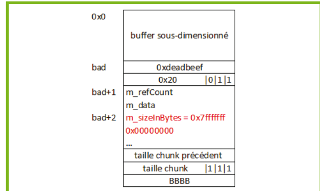
Fig. 6 : Réécriture de la taille du WTF::ArrayBuffer .
