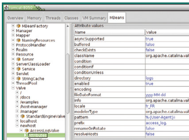
Fig.5 : Configuration d'un AccessLoggerValve permettant le dépôt de contenu via le user-agent.
