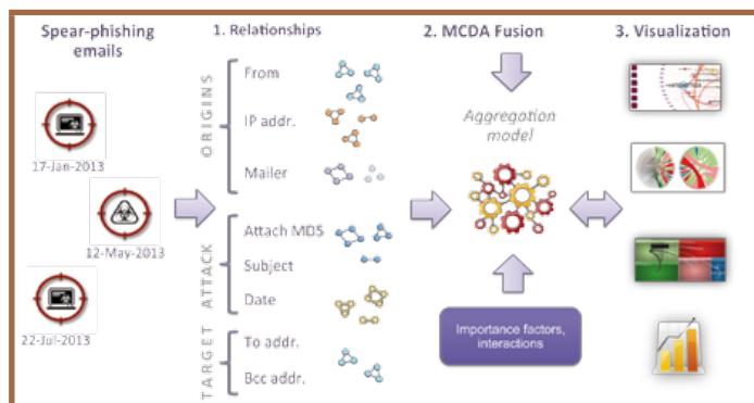
Fig. 2 : Illustration de l'approche TRIAGE qui combine des techniques de fouille de données et de visualisation afin de faciliter l'investigation de campagnes de cyberattaques.
