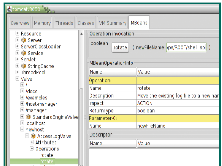
Fig.6 : Déplacement du fichier de log dans l'arborescence sur serveur web.
