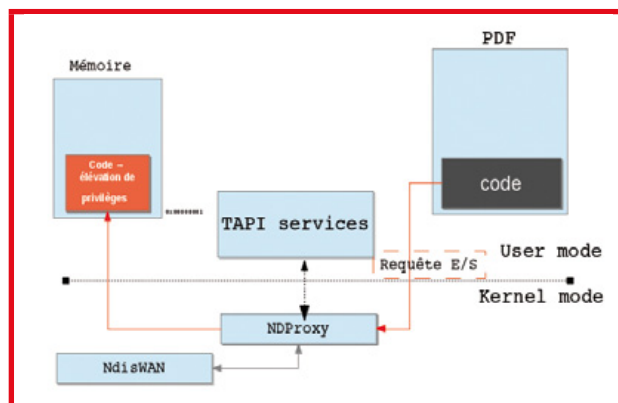
Fig. 0 : Description globale de la vulnérabilité.
