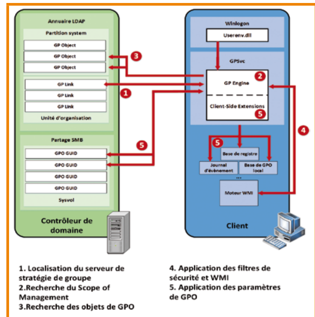
Fig. 2 : Schématisation de l'architecture supportant le mécanisme de stratégie de groupe.
