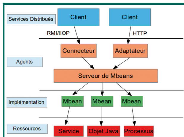
Fig.1 : Schéma d'architecture de l'API JMX.
