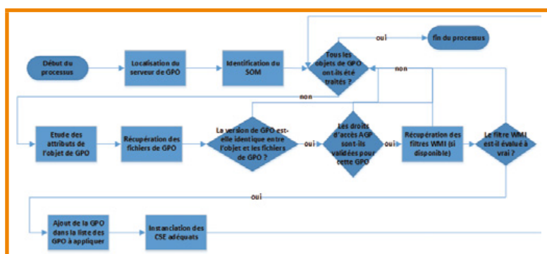
Fig. 3 : Étapes d'application des stratégies de groupes.
