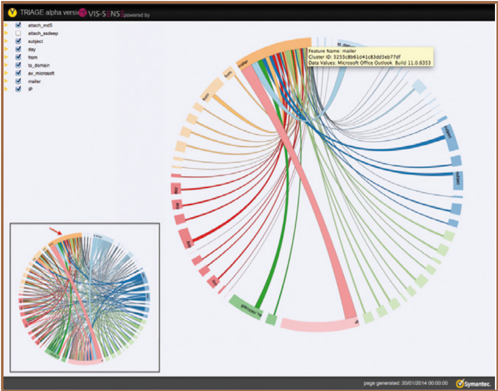
Fig. 8 : La campagne d'attaques APT1/CommentCrew, visualisée ici à l'aide d'un diagramme en cordes généré sur les groupes d'e-mails partageant une caractéristique commune (même adresse From, sujet similaire, etc.).
