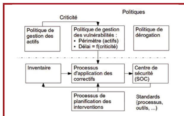
Fig. 1 : La gestion des vulnérabilités pour les NULS.
