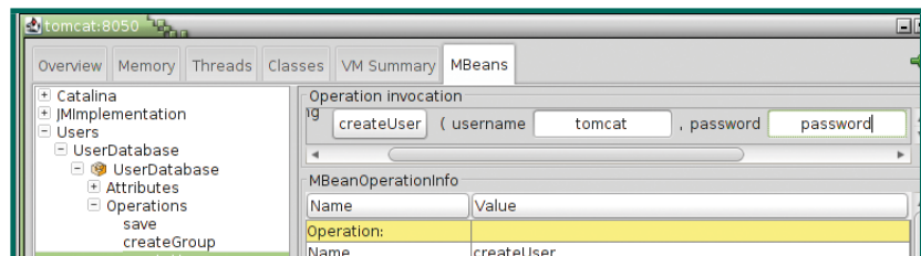
Fig. 2 : Création de l'utilisateur tomcat.
