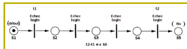
Fig. 5 : Quatre échecs d'authentification en une minute.
