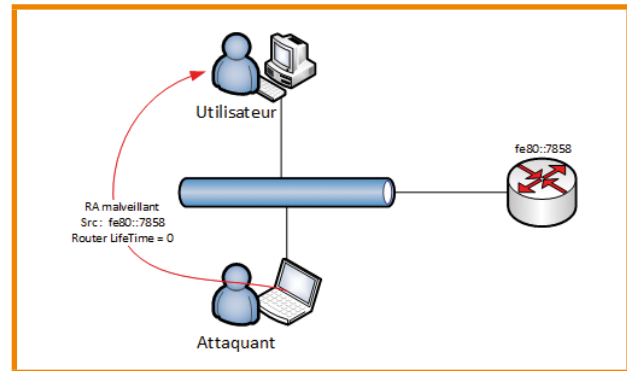
Fig. 2 : Schéma d'attaque DOS en utilisant les messages RA.
