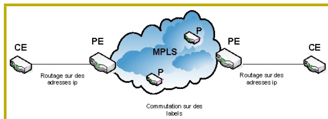
Figure 1 : Réseau MPLS
