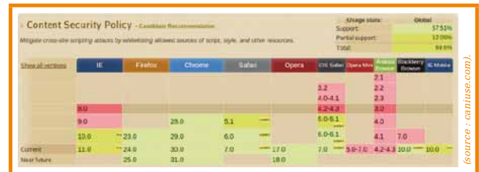
Fig. 1 : Support de CSP dans les différents navigateurs
