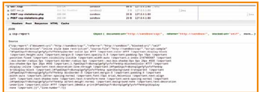
Fig. 2 : Exemple de violation CSP.
