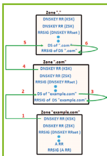
Fig. 2 : Un exemple de comment une chaîne de confiance est établie.
