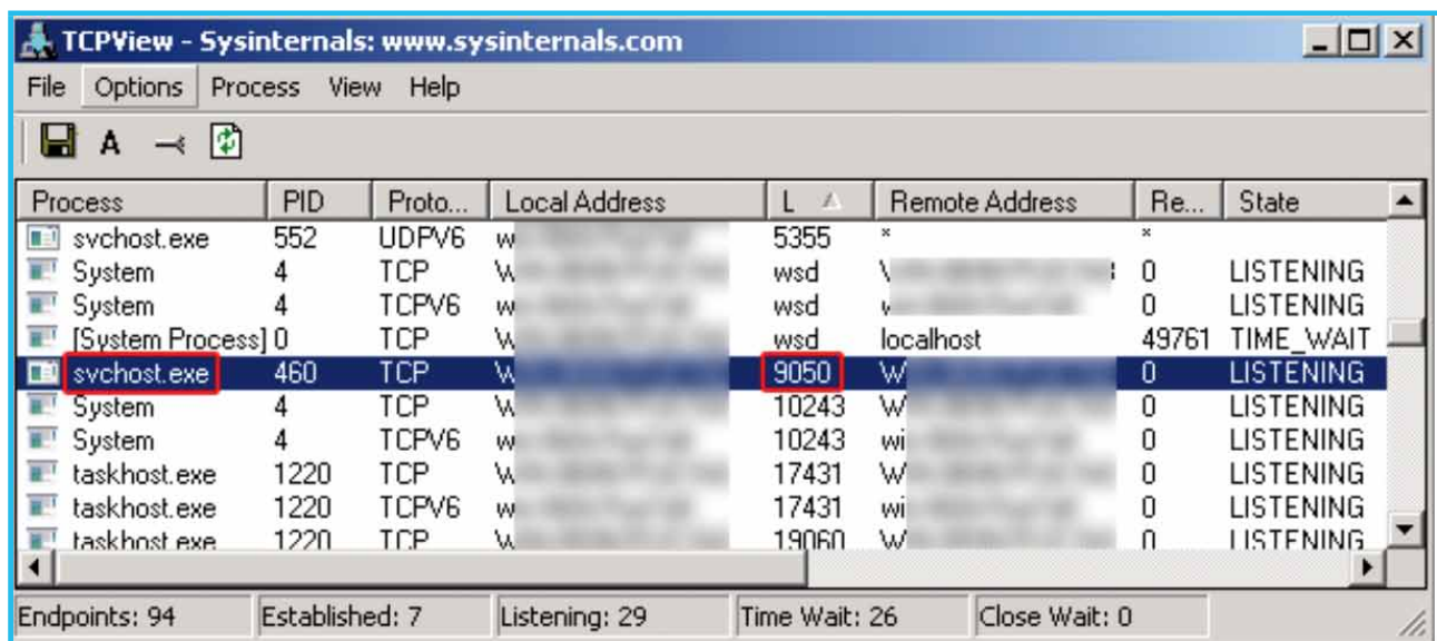
Fig. 5 : Port ouvert par le proxy Tor une fois injecté dans le process « svchost.exe ».
