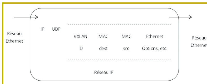
Figure 6 : Encapsulation de trames VXLAN dans UDP.
