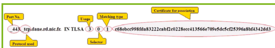
Fig. 4 : Différents champs de TLSA.
