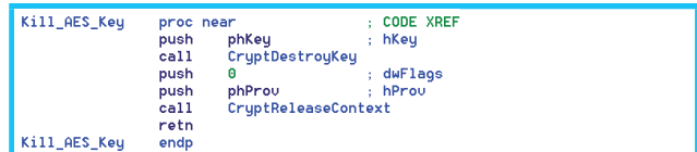
Figure 12 : Destruction de la clé AES
