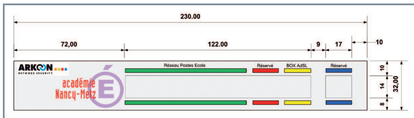
Figure 8 : Plastron d'habillage du boîtier
