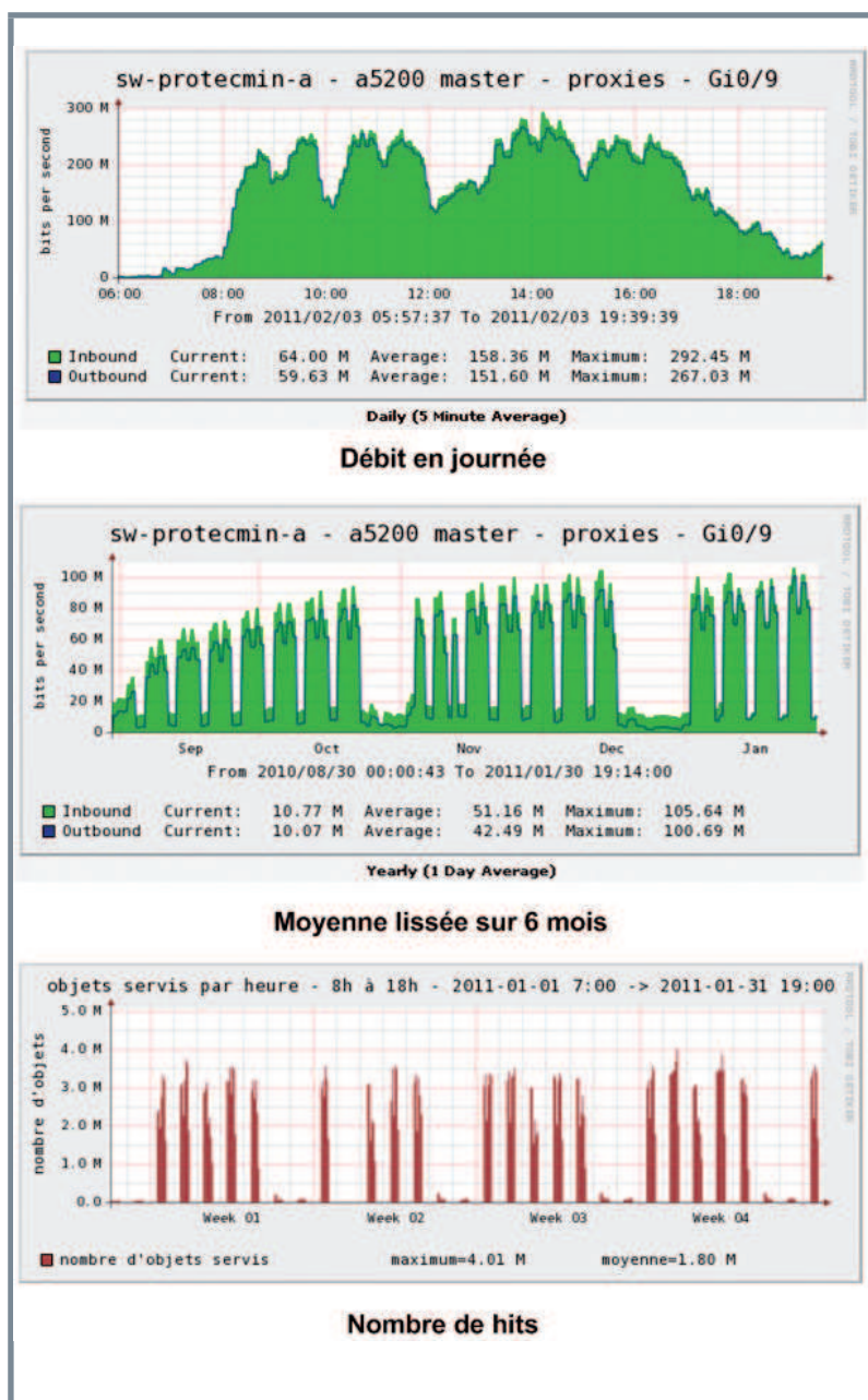
Figure 10 : Débit de la plateforme
