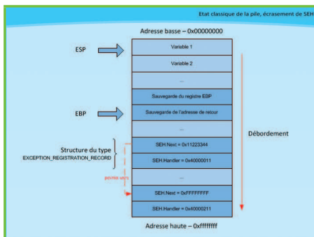
Cas classique d'une réécriture d'un gestionnaire d'exception SEH dans la pile
