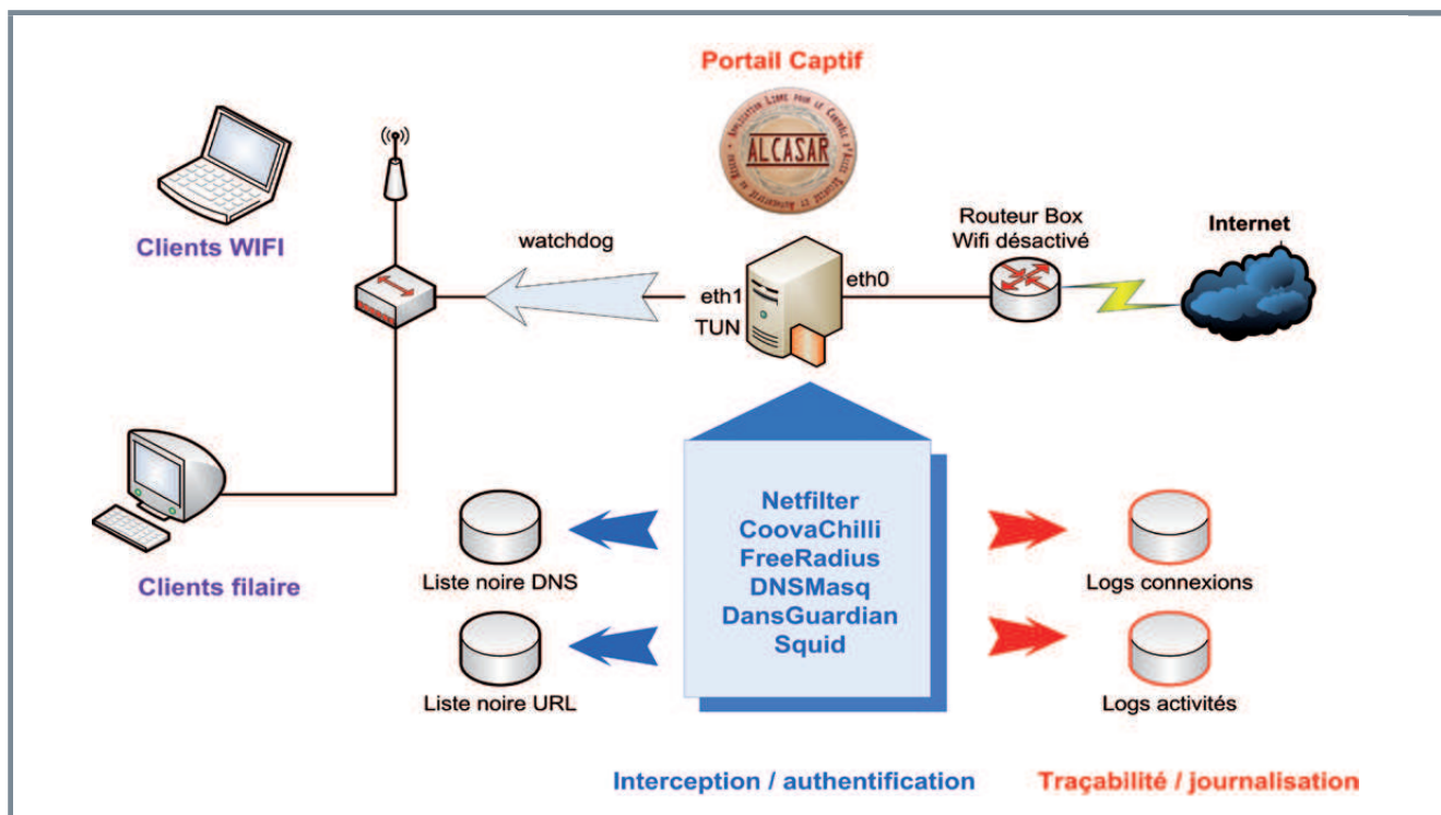
Fig 2 : Schéma d'architecture Alcasar
