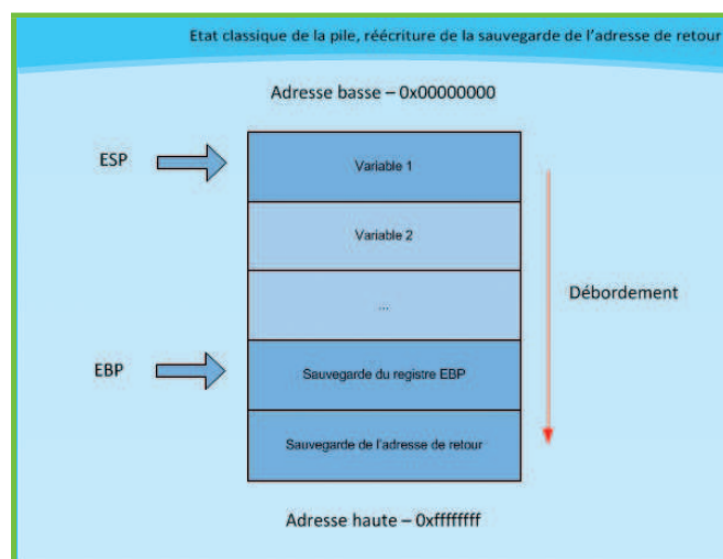
Cas classique d'un débordement de tampon dans la pile
