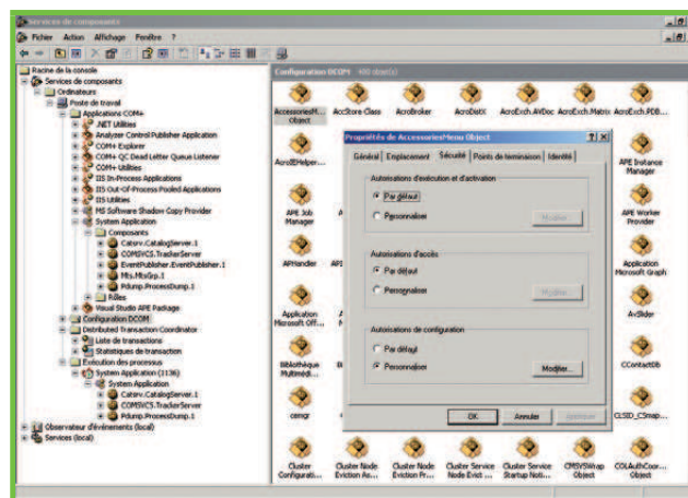
Figure 2 : DCOMCNFG.EXE en action
