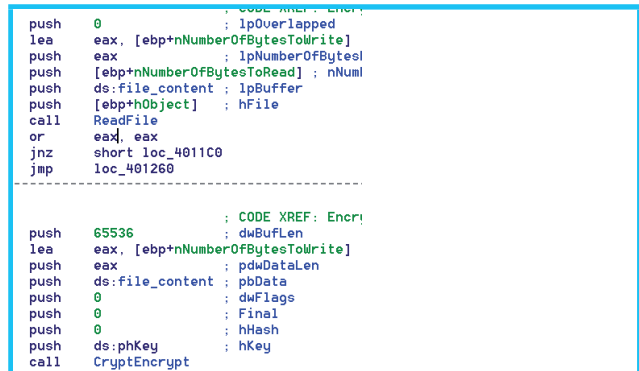
Figure 11 : Routine de chiffrement de Gpcode
