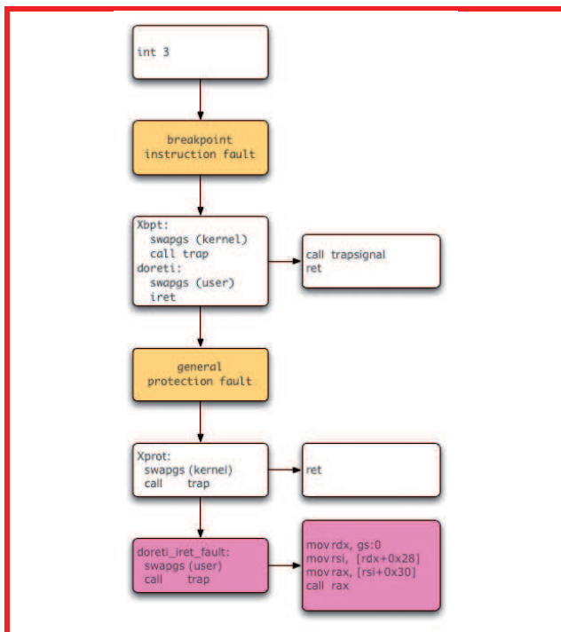
Flot d'exécution, de l'interruption à la vulnérabilité
