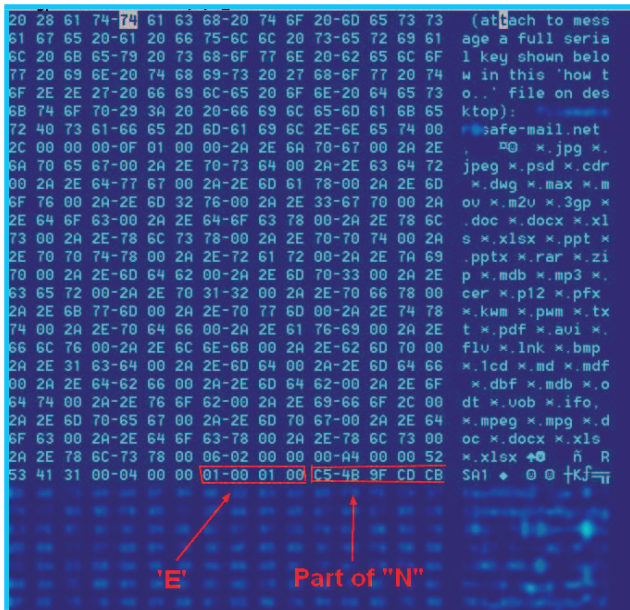
Figure 8 : Fichier de configuration décodé
