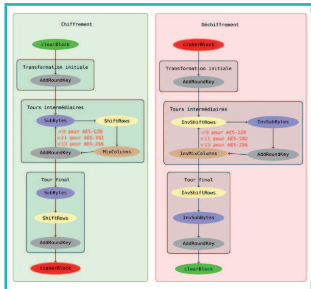
Fig. 1 : Les processus de chiffrement et de déchiffrement de l'AES
