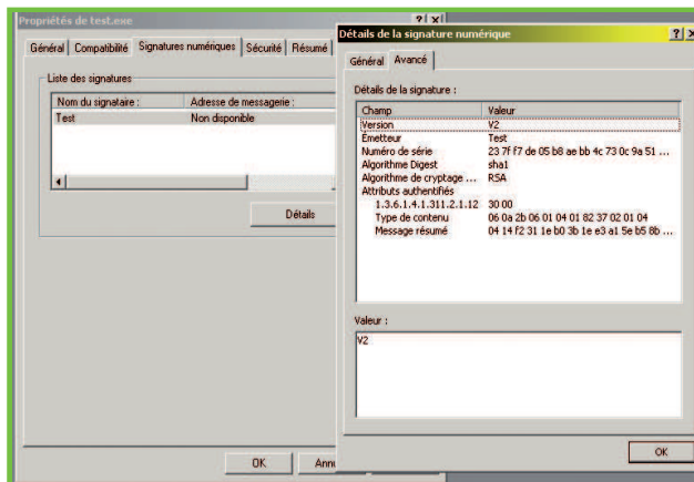
Figure 1 : Fichier test.exe signé avec un certificat embarqué
