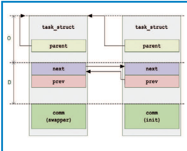
Fig. 2 : Relations entre les champs de task_struct
