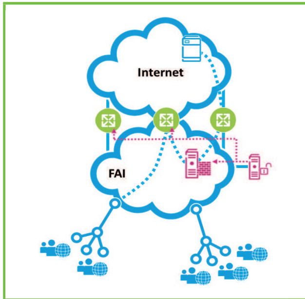
Fig. 3 : Le principe est similaire à l'exemple précédent, sauf que le routeur ne détruit pas le trafic mais le redirige vers un relais applicatif. Le trafic « autorisé » sortant du relais contourne les routeurs filtrants. Cette image n'est qu'un exemple, il existe de nombreuses variantes de cette architecture (injection de route à un autre niveau du réseau, par exemple au niveau de l'accès ou de l'agrégation, utilisation de tunnels de type GRE ou L2TPv3, etc.). Cette approche est souvent une réplique des mécanismes avancés de filtrage des attaques par déni de service.
