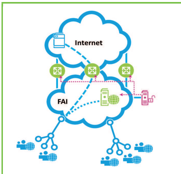
Fig. 2 : Réseau d'opérateur avec les clients (au bas de l'image) connectés via un réseau d'accès avec un serveur DNS récurif et des routeurs de bordure (peering et transit). La plate-forme de gestion du filtrage annonce via BGP les préfixes/IP à filtrer et publie les zones à filtrer au niveau DNS. Les routeurs et les serveurs DNS agissent comme un trou noir pour les sites à filtrer.
