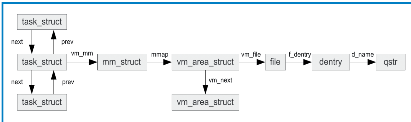
Fig. 1 : Relations entre les structures noyau
