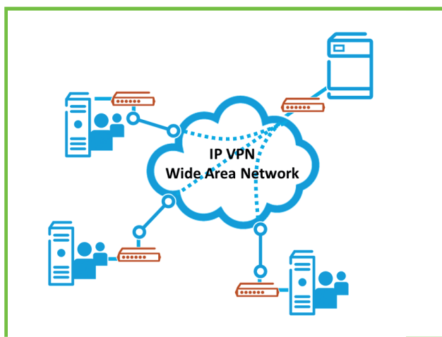
Fig. 1 : Réseau privé virtuel de type IP VPN hub&spokes avec sur chaque site un équipement DPI pour, par exemple, accélérer les transferts de fichiers ou l'accès terminal.
