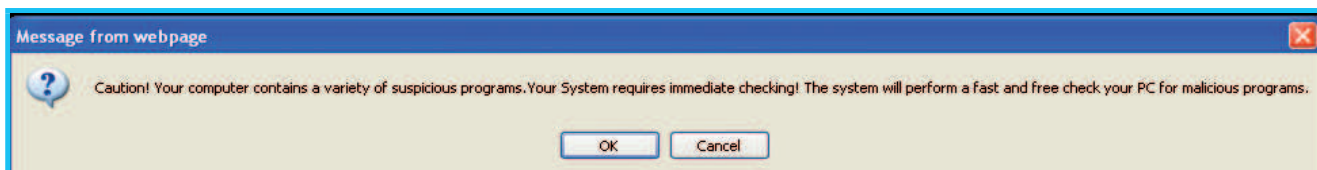
Figure 6 : Alerte d'infection
