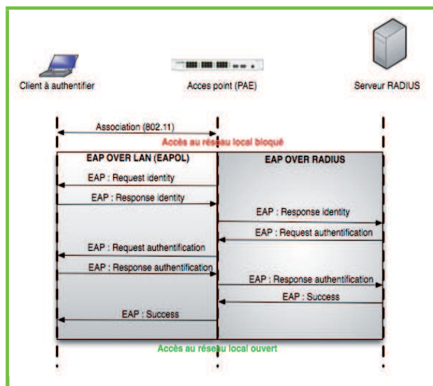
Figure 3 : Schéma d'échange EAP dans le Wi-Fi
