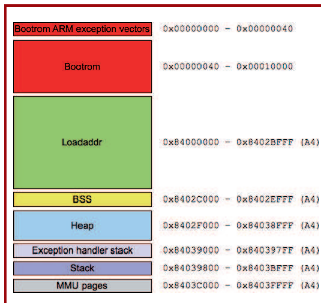
Fig. 4 : Carte mémoire de la bootrom
