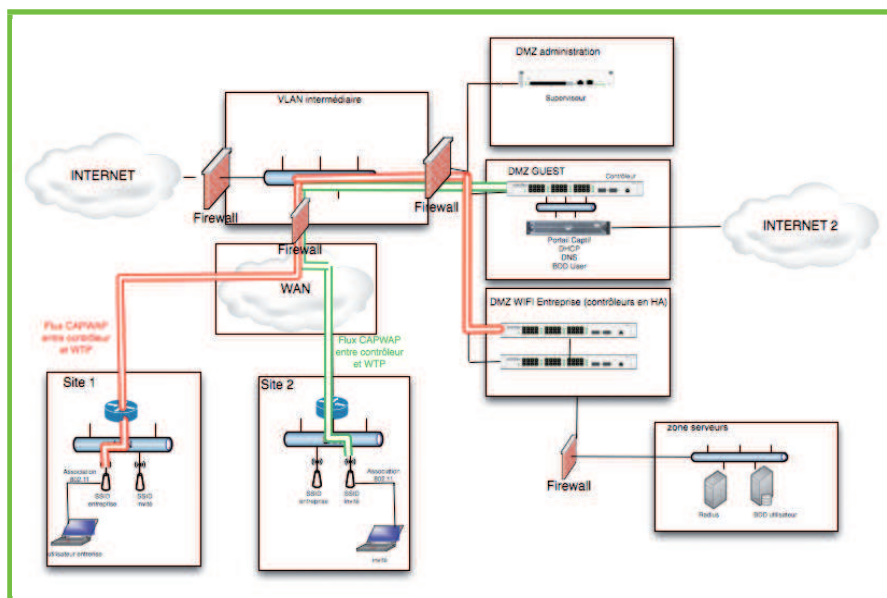
Figure 4 : Schéma simplifié d'architecture sécurisée
