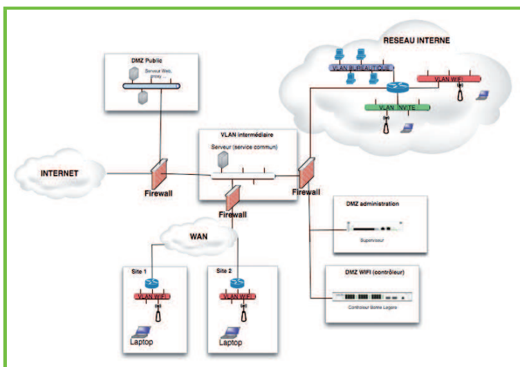
Figure 1 : Schéma simplifié d'architecture centralisée multisites
