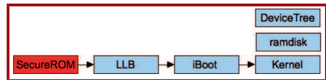
Fig. 2 : Chaîne de démarrage iOS en mode recovery
