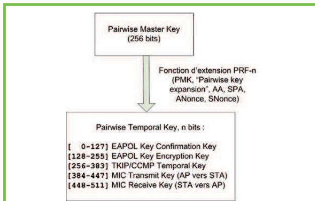
Schéma 1a : 4-way handshake
