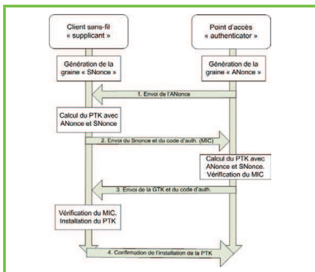
Schéma 1b : Dérivation de la PTK
