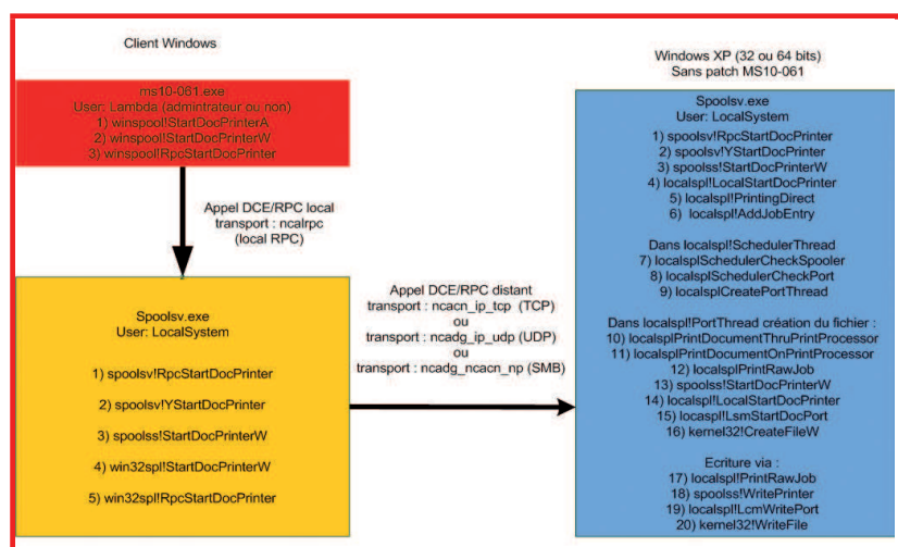
Interactions entre les 2 spoolers et création du fichier sur le Windows distant
