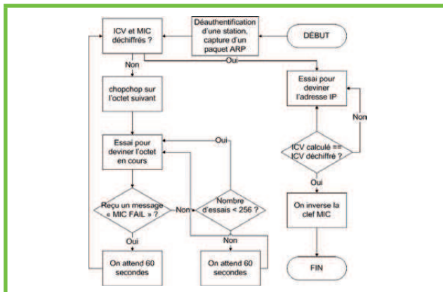
Schéma 1c : processus de déchiffrement
