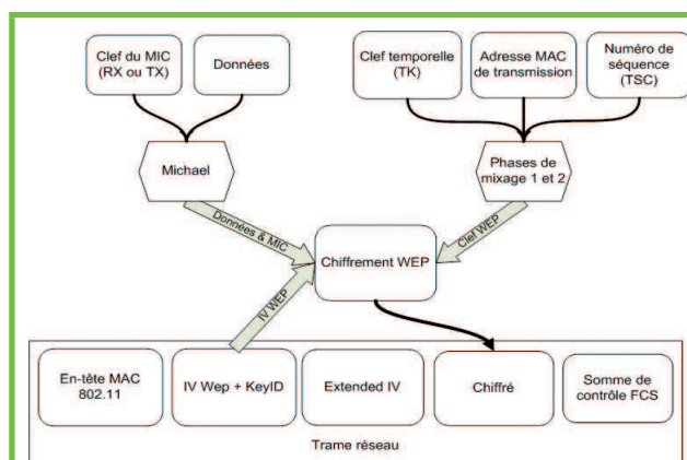
Fig. 1 : Trame chiffrée avec TKIP
