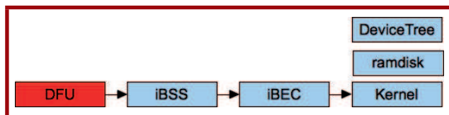
Fig. 3 : Chaîne de démarrage iOS en mode DFU
