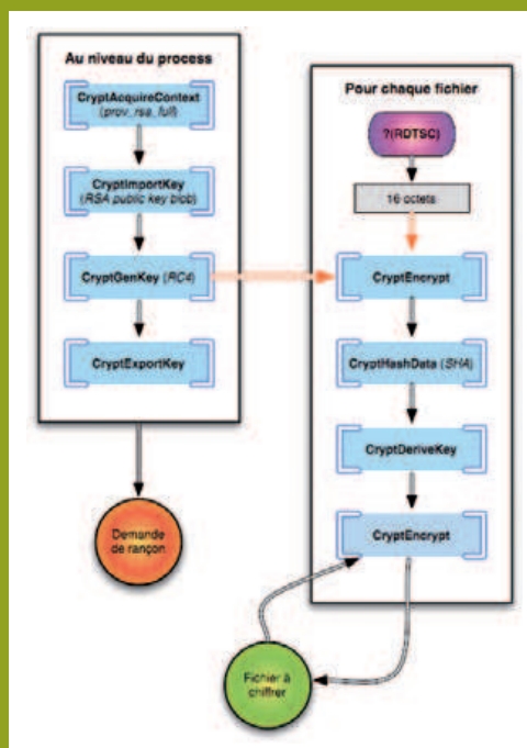
14 Cryptosystème hybride, Gpcode.ak
