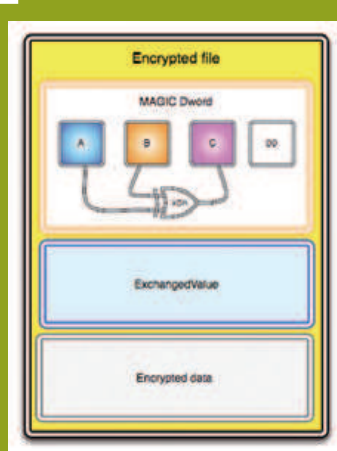
8 En-tête d'un fichier chiffré avec Gpcode.ab
