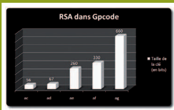
10 Évolution de la taille de la clé RSA
