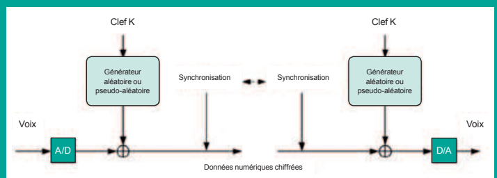
4 Système cryptophonique numérique à synchronisation additionnelle.
