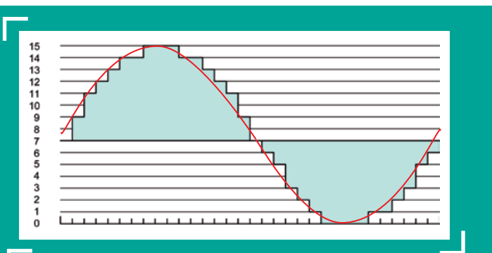
Échantillonnage d'un signal analogique (méthode PCM ; les lignes verticales représentent les valeurs F(t) pour des instants réguliers t ).
