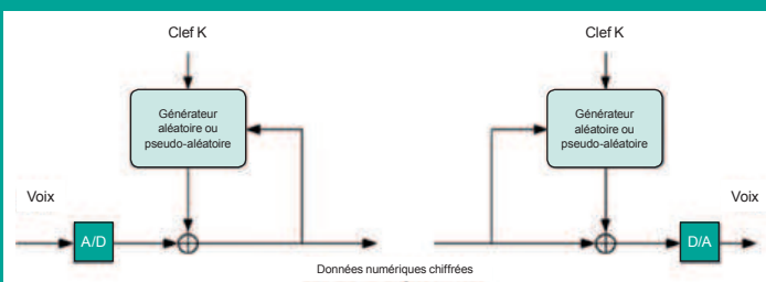
3 Système cryptophonique numérique avec autoclave sur le chiffré
