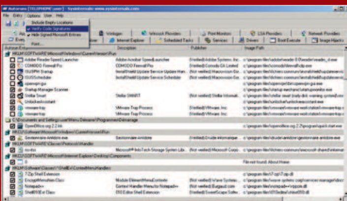
6 Outil Autoruns
