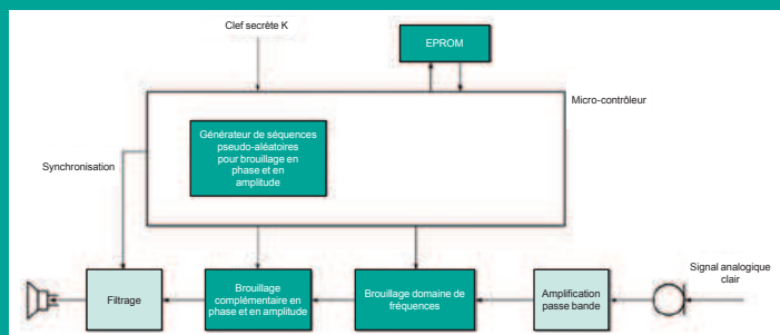
5 Système de brouillage vocal analogique militaire chinois (schéma simplifié sans la partie électronique).
