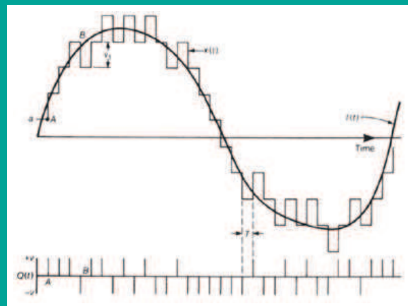
2 Principe de modulation linéaire delta
