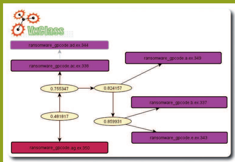
15 Indices de similarité dans VxClass
